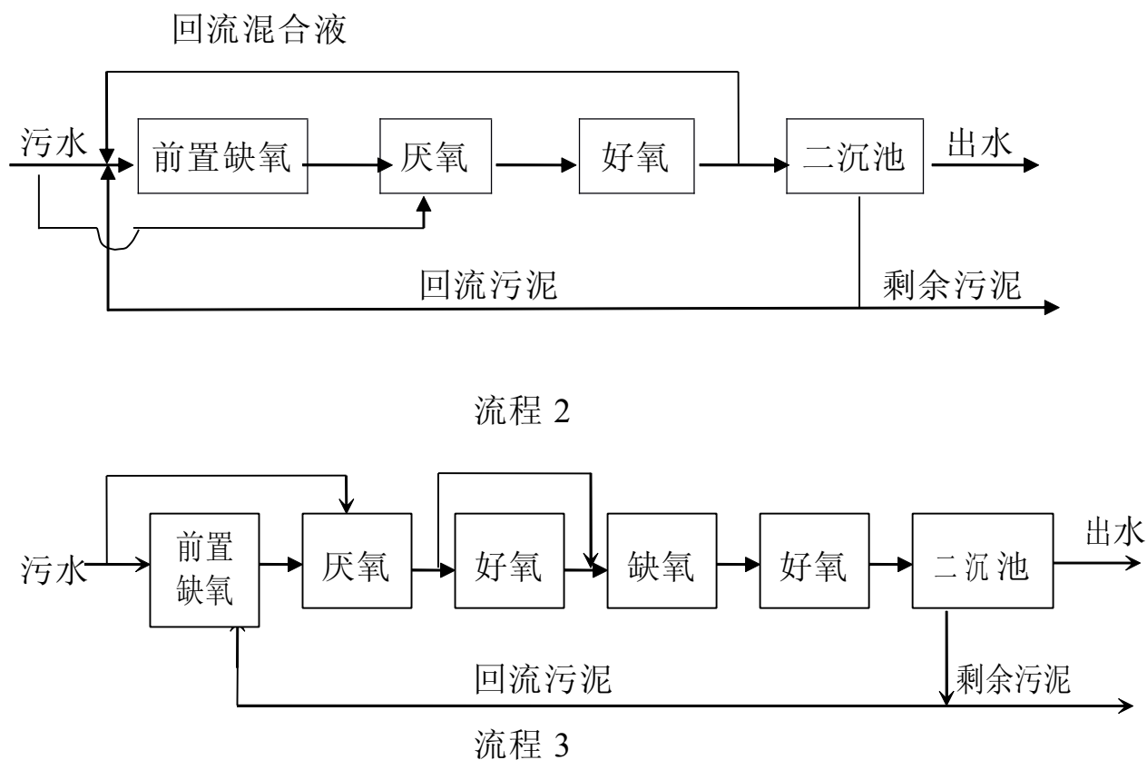
图 3 一些变型的工艺流程
